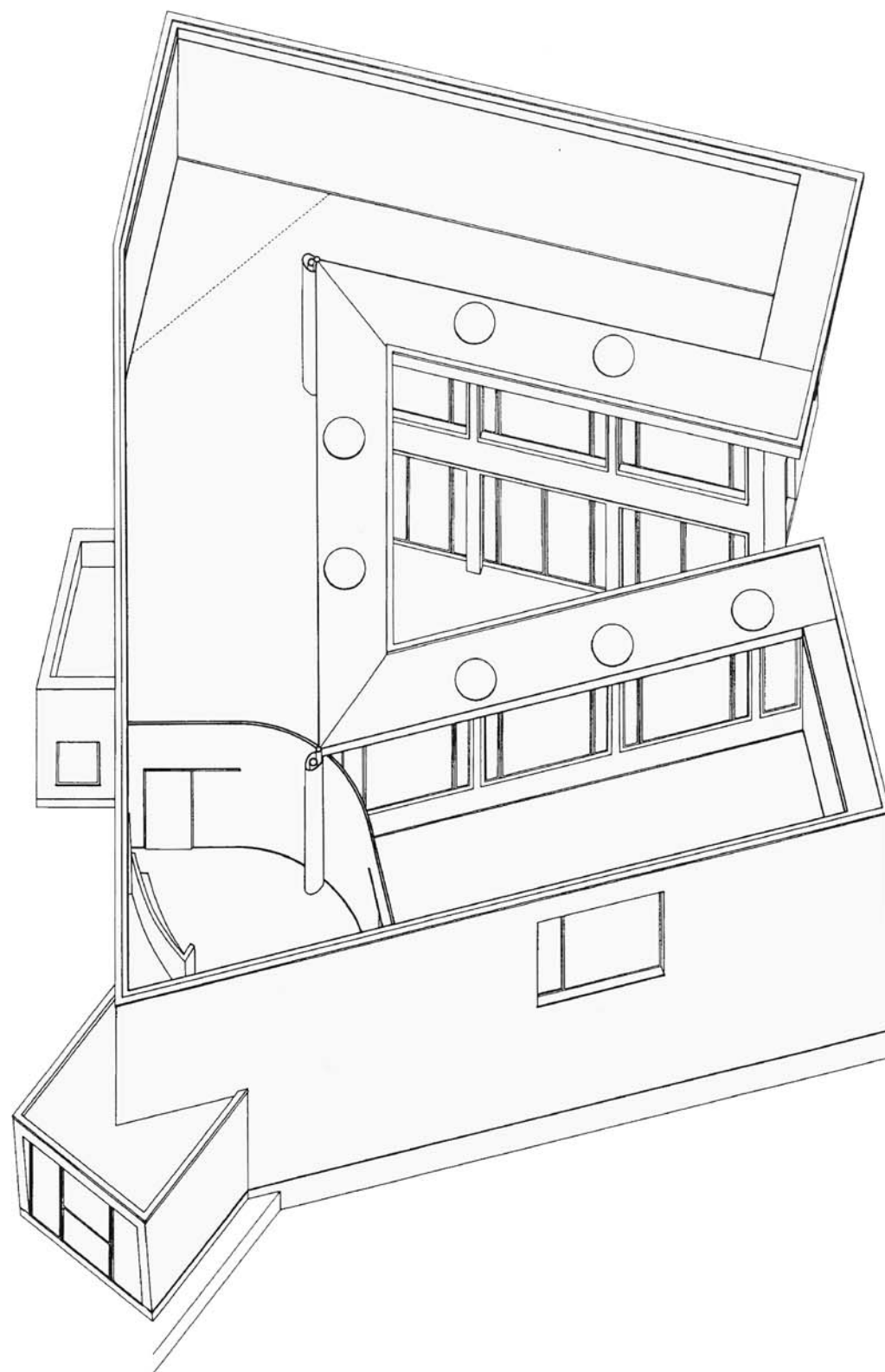
spaccato assonometrico
