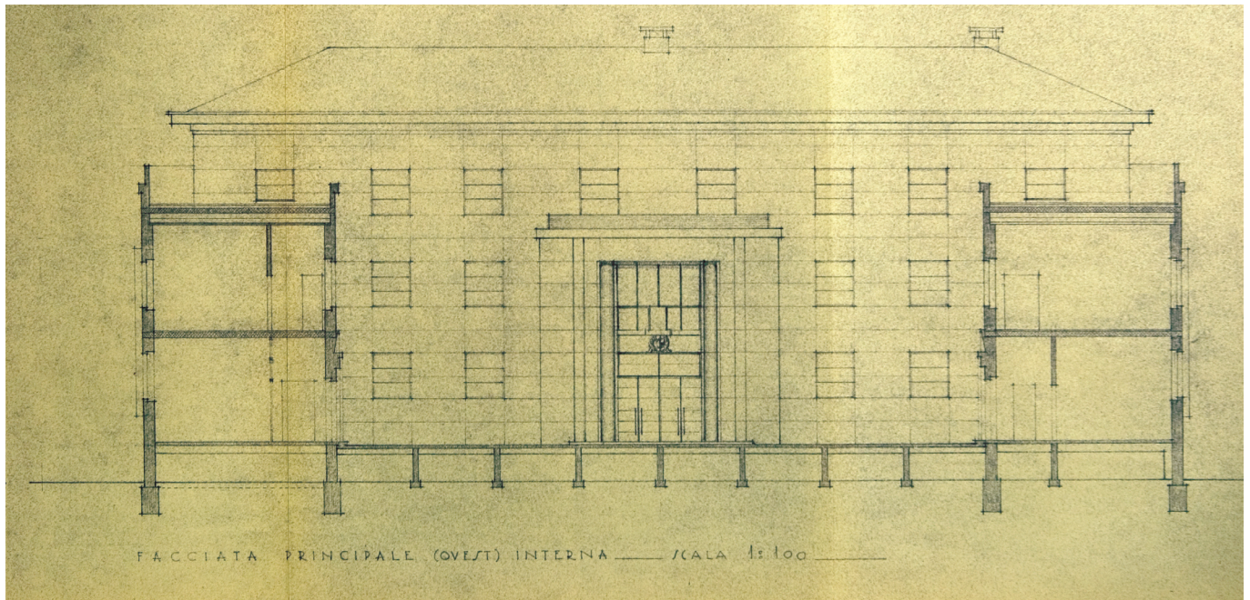
Sezione sulla corte d'onore.
