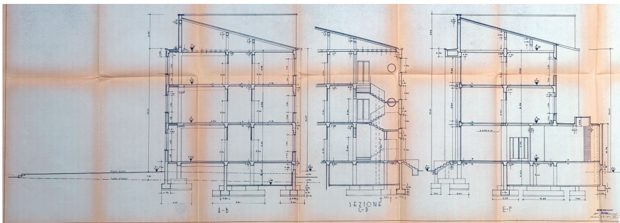
Sezioni.
