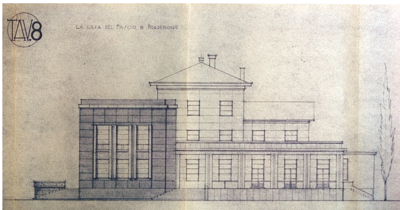
Il prospetto del fianco su Viale Marconi mostra la grande finestra sull'ala minore della Gil e il portico laterale con ordine minore.
