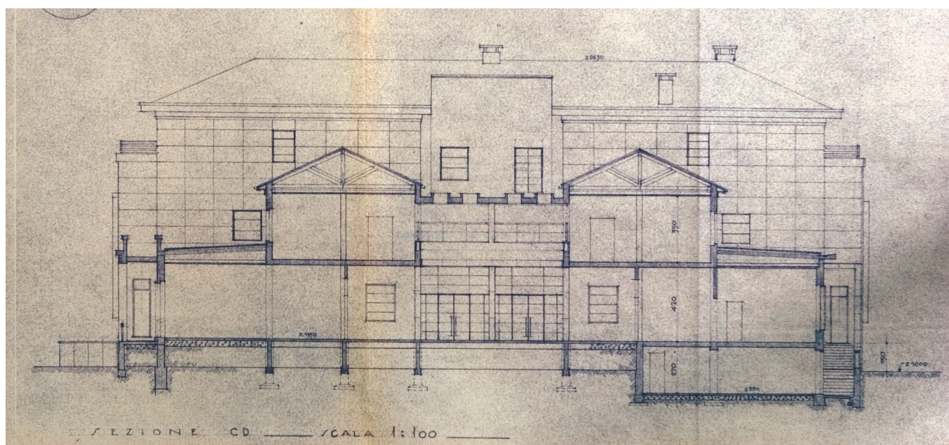
Sezione trasversale sulla sala delle adunanze. Si nota come nella prima versione del progetto fosse previsto un portico in ordine minore solo su via Marconi.
