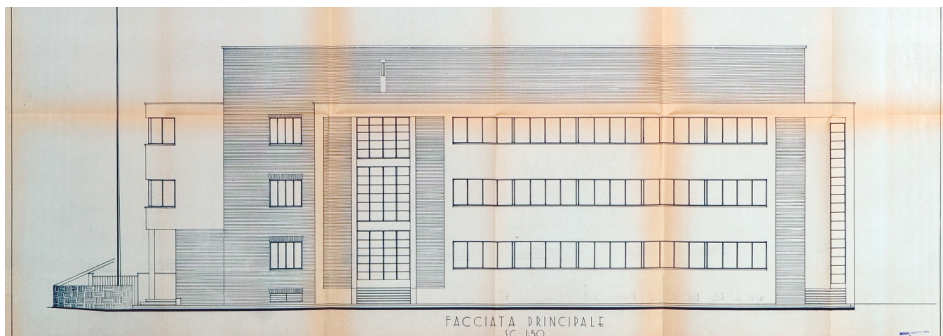
La facciata principale è studiata con la contrapposizione di tre piani: il primo intonacato, il secondo rivestito in klinker e il terzo nuovamente intonacato.
