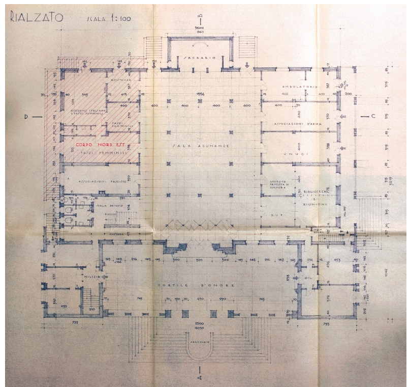
Pianta del piano rialzato nella prima versione 1939.
