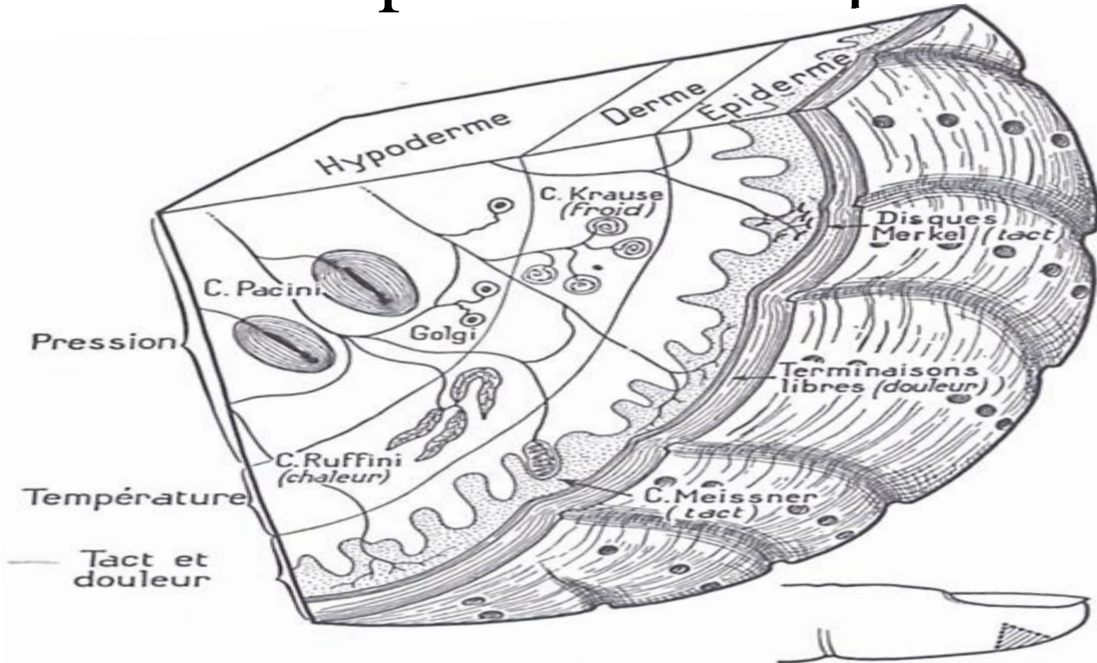
FIG. 23. — Coupe schématique de la peau du doigt. Situation des différents types d'exorécepteurs.
